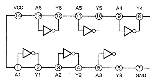
IC306 74HCU04
